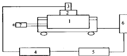
1—振动台；2—试样；3—传感器；4—电荷放大器； 5—振动控制仪；6—功率放大器；7—风机
